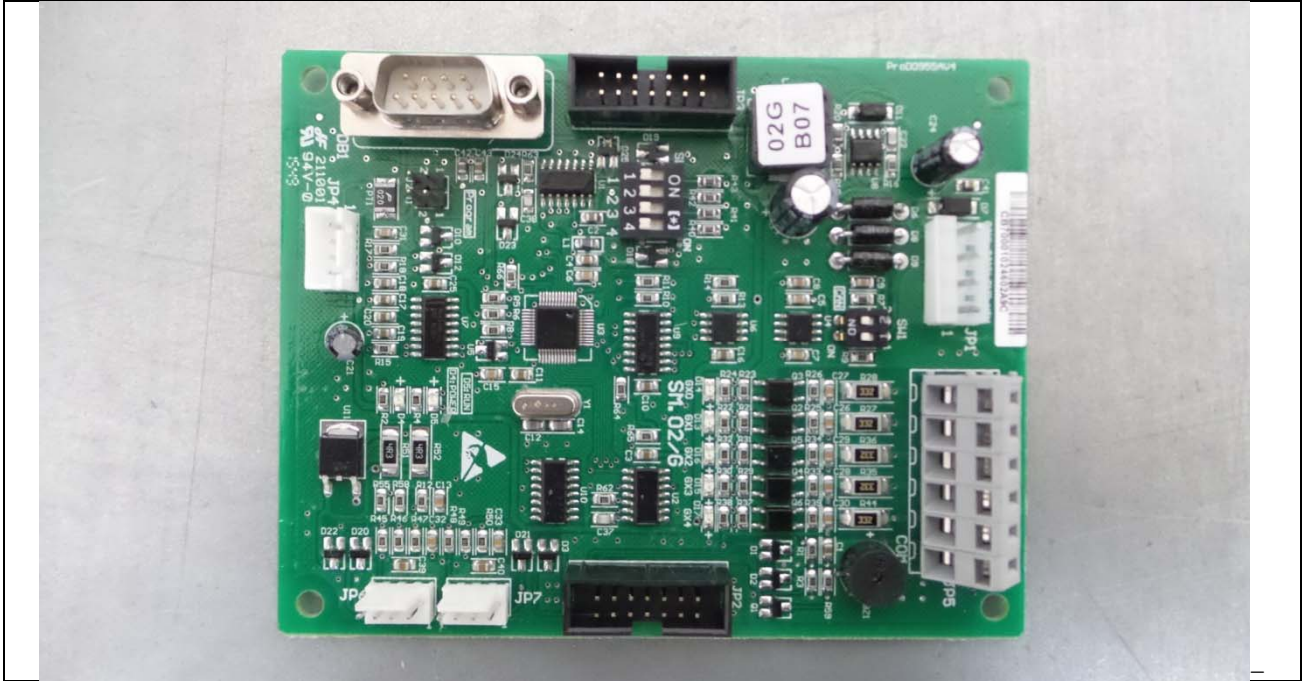
인버터_내부PCB_정면
