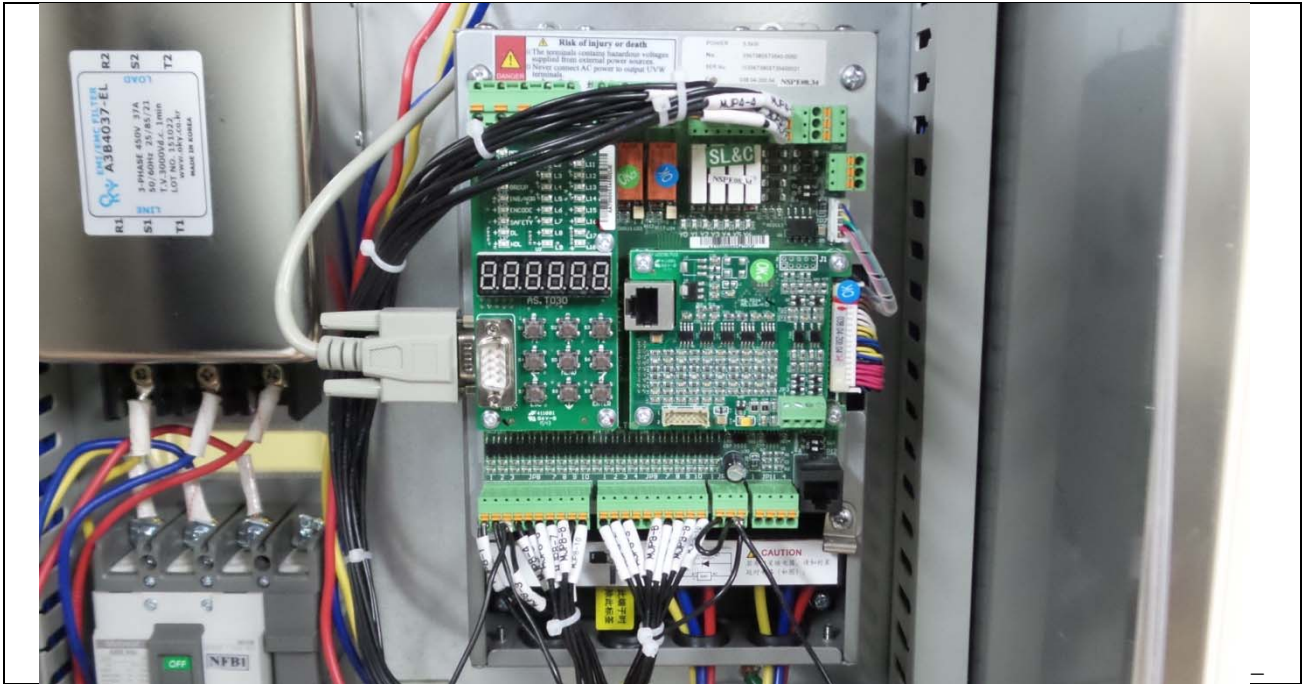
인버터 내부
